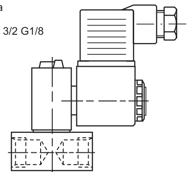
Zawór rozdzielający 3/2 G1/8 NZ
